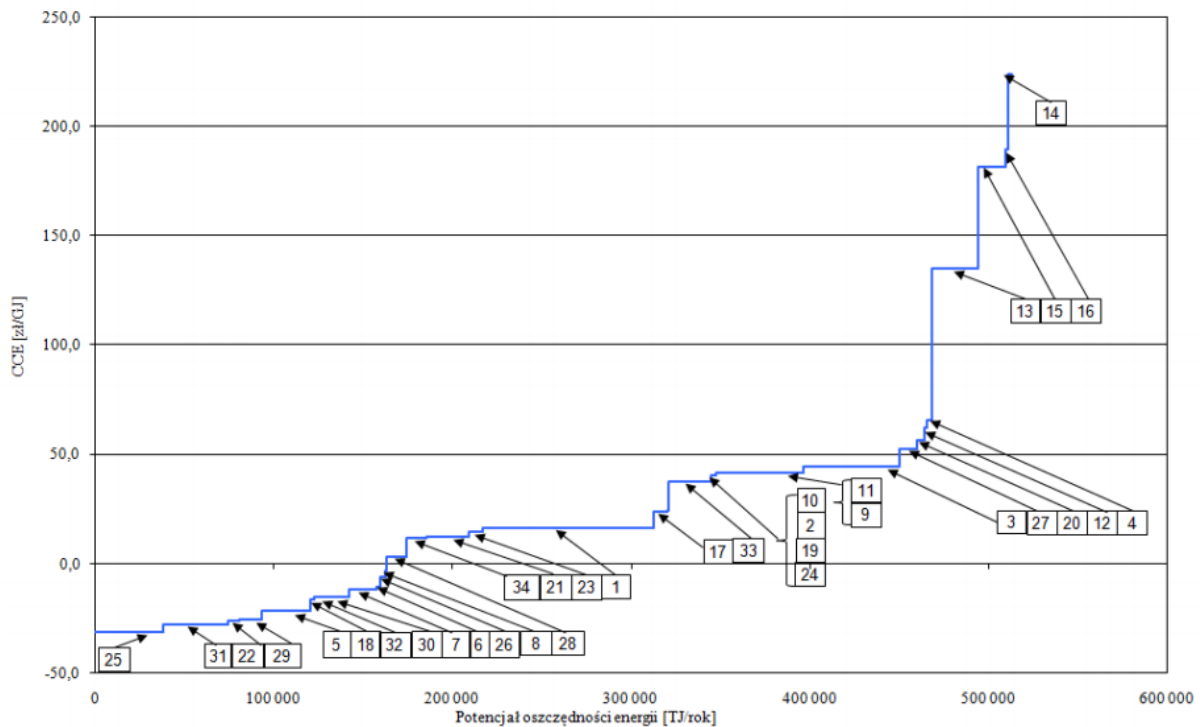
Rysunek 16. Potencjał oszczędności energii w budynkach w Polsce. Objasnienia oznaczeń przedstawia Tabela 31
